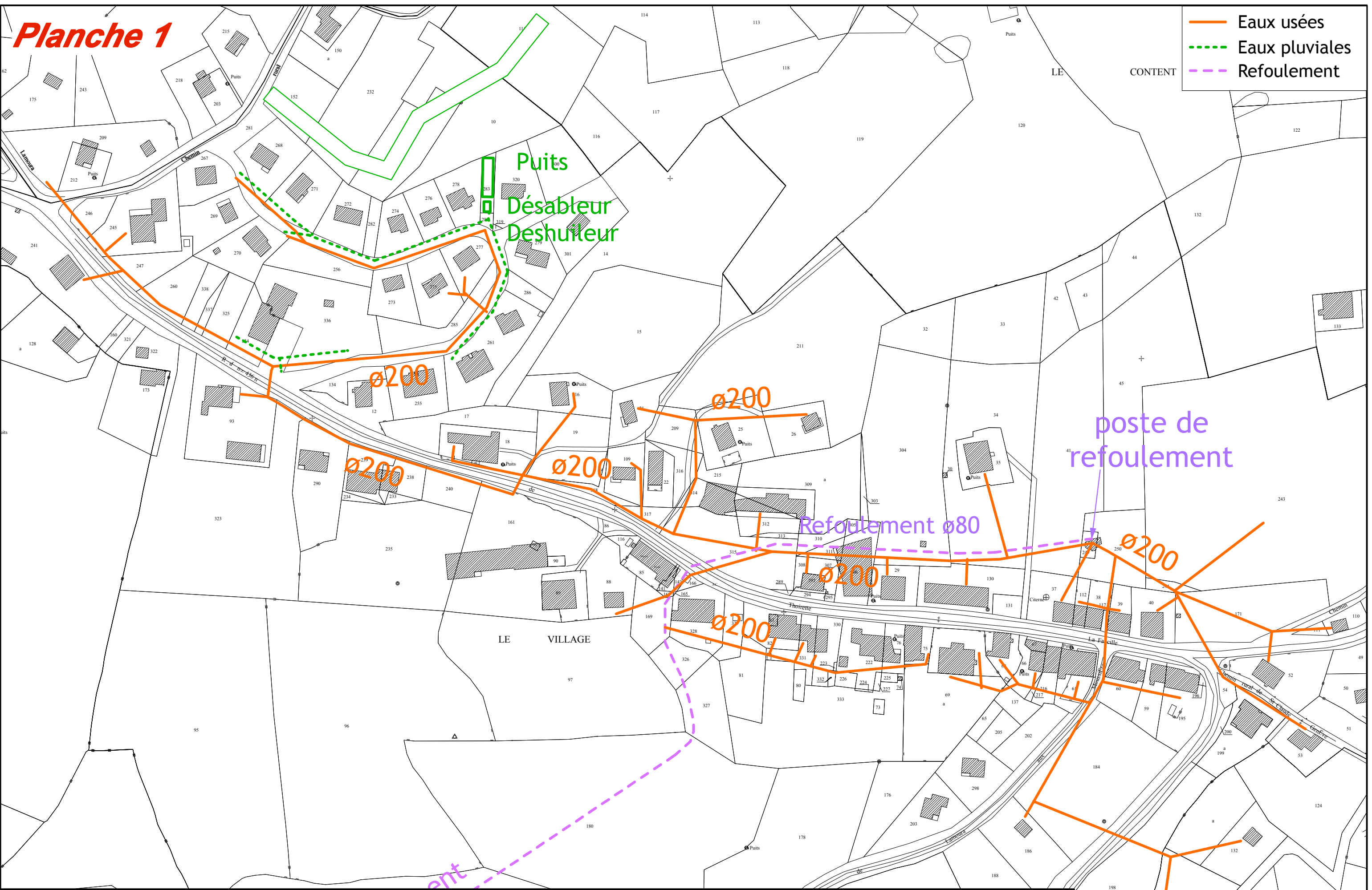
Commune de LAJOUX - Réseaux d'assainissement d'après les plans dessinés par B&R Environnement en Juin 2003 - Planche 1 - 1/2000
